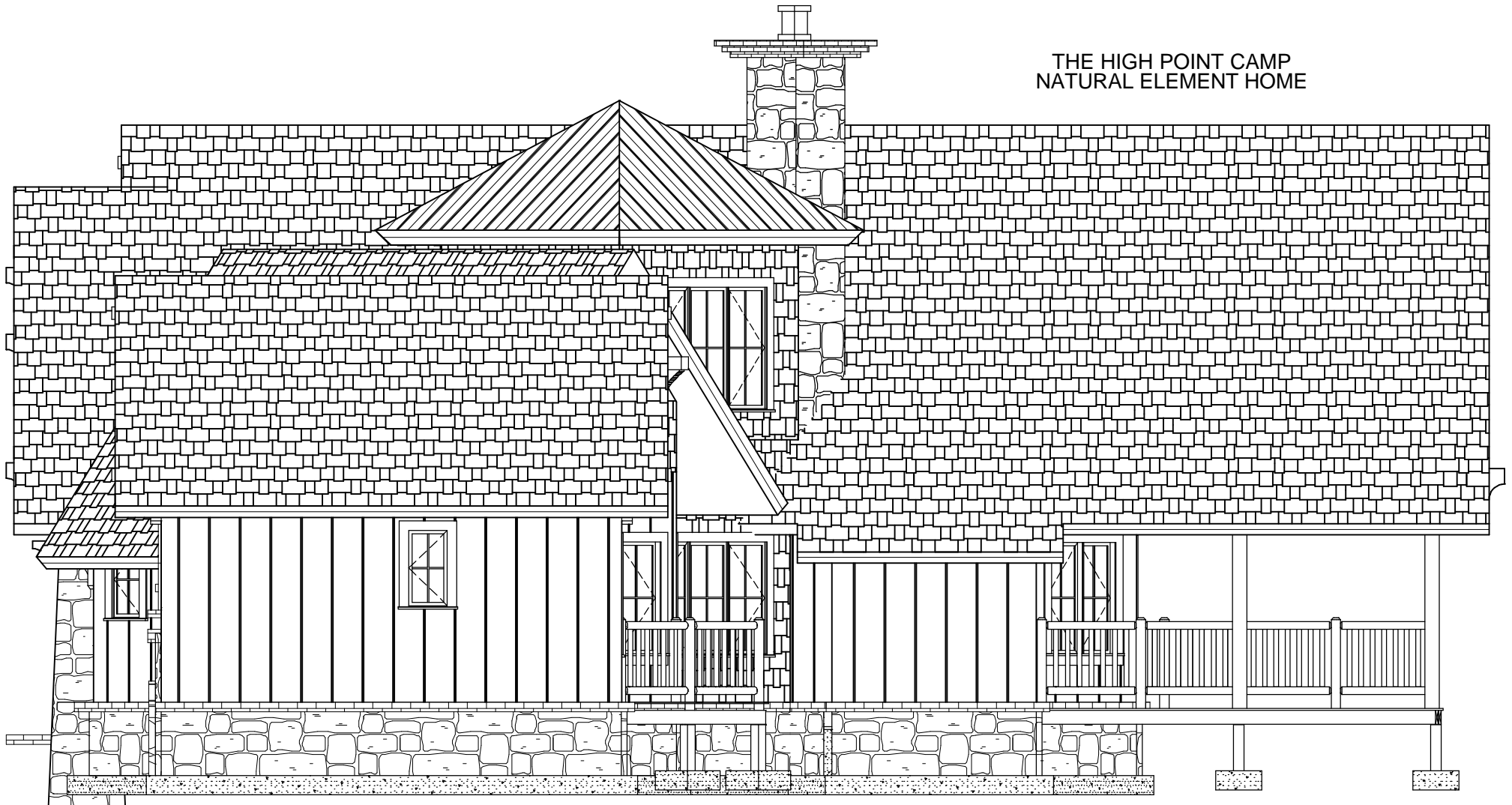
RIGHT ELEVATION
