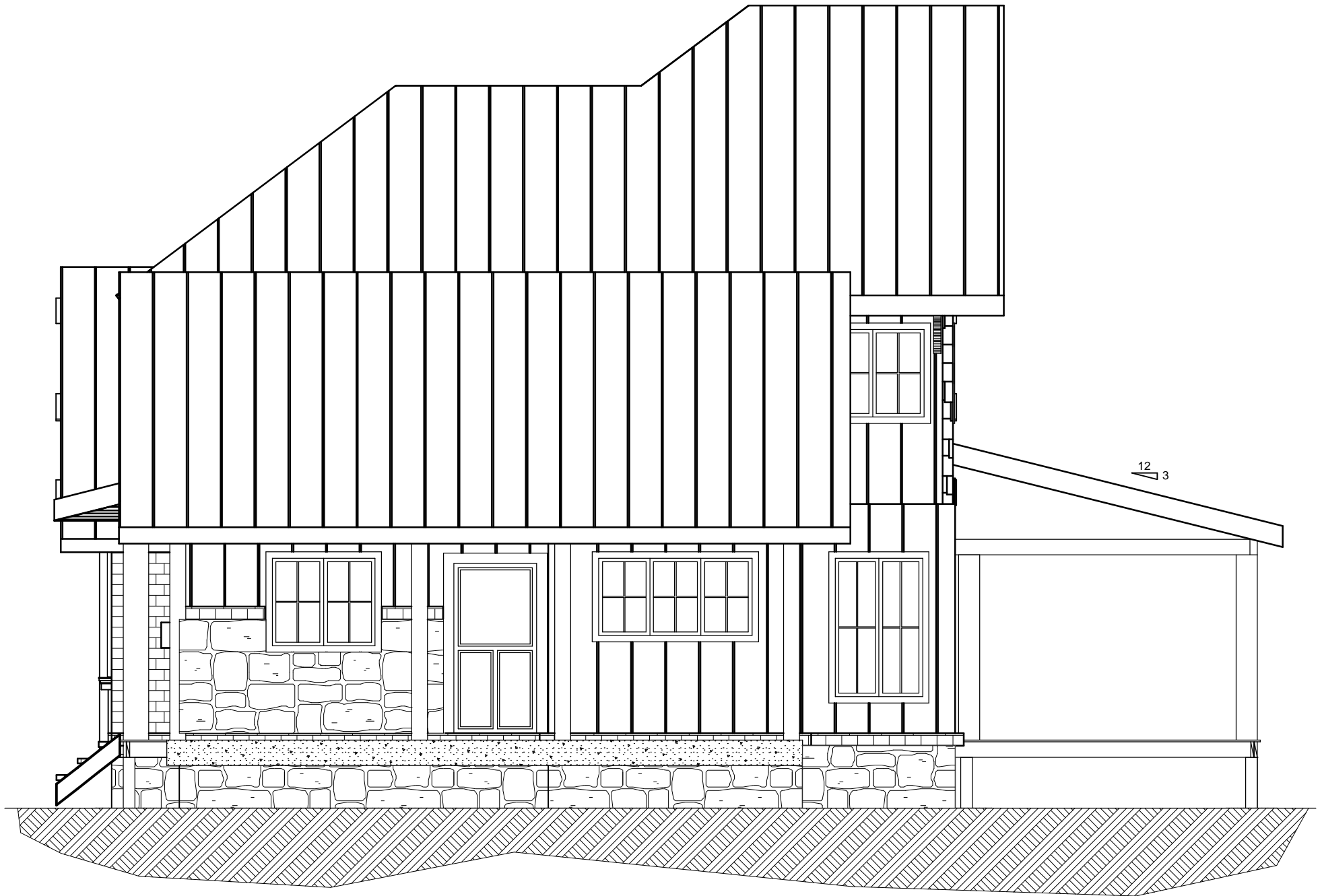
RIGHT ELEVATION
