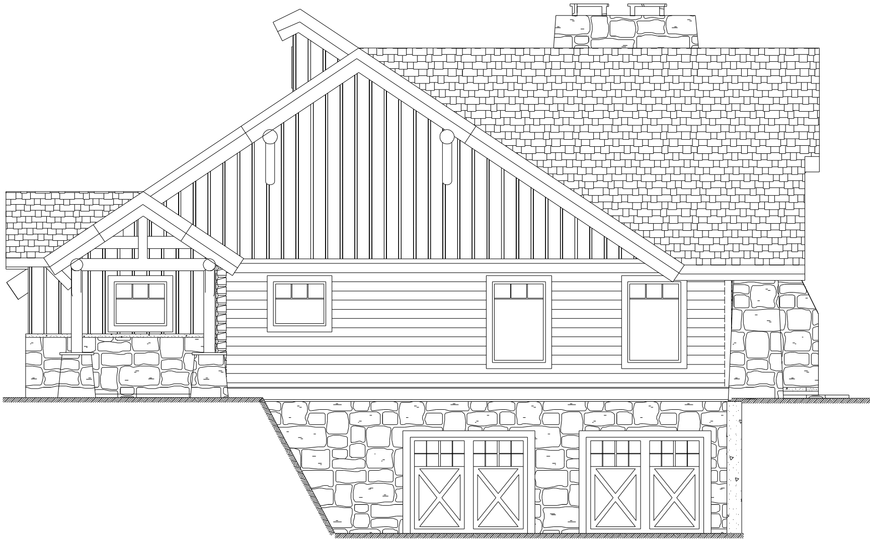
RIGHT ELEVATION
